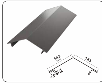
COAMĂ RETRO
