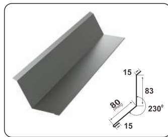
BORDURĂ LA PERETE
