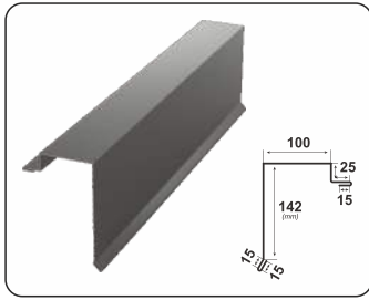
BORDURĂ FRONTON RETRO
