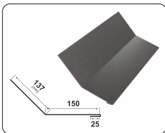
RUPERE PANTĂ CONCAVĂ
