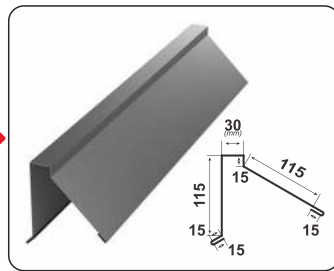
SEMICOAMĂ UNGHIULARĂ
