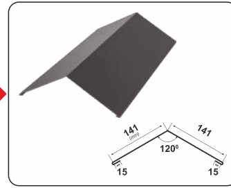
COAMĂ UNGHIULARĂ
