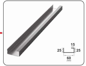
SUPORT COAMĂ
