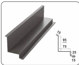
BORDURĂ LA PERETE LATERALĂ RETRO
