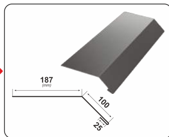
RUPERE PANTĂ CONVEXĂ
