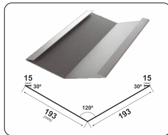
DOLIE RETRO
