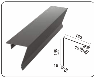
SEMICOAMĂ RETRO
