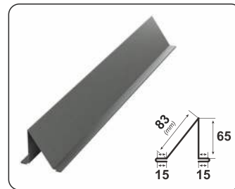
OPRITOR ZAPADĂ
