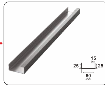
SUPORT COAMĂ
