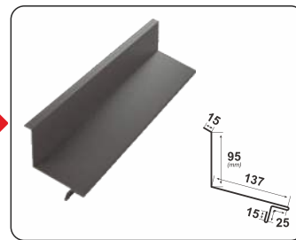
BORDURĂ LA PERETE ORIZONTALĂ RETRO
