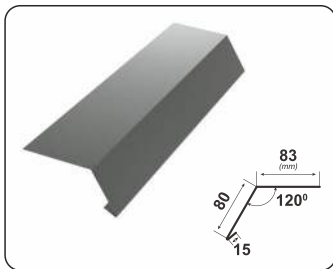
BORDURĂ STREĂȘINĂ
